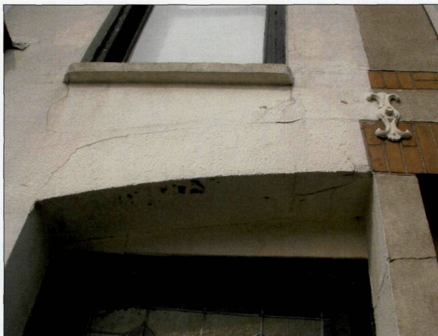
Foto 5: Diverse scheuren met name in de toog en de penant bij voorgevel nr. 42.
