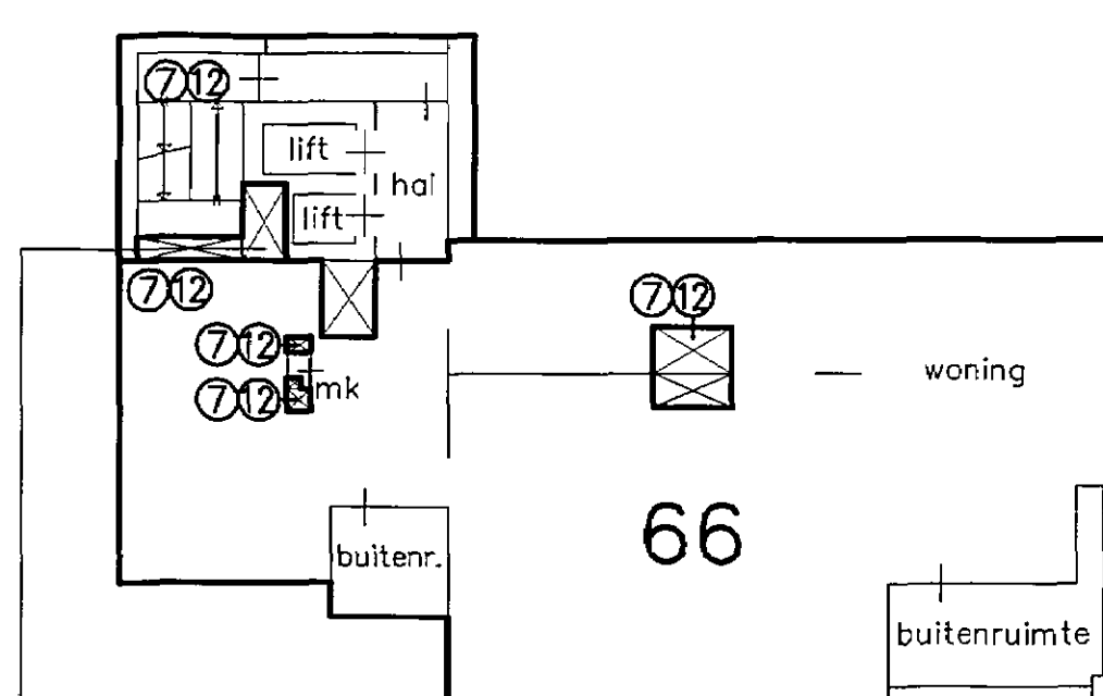
Bouwnr. 49 schachten voor algemeen gebruik woningen + comm.ruimten
