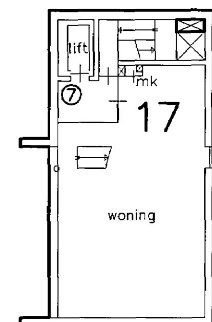
8e verdieping Schaal 1 a 200
