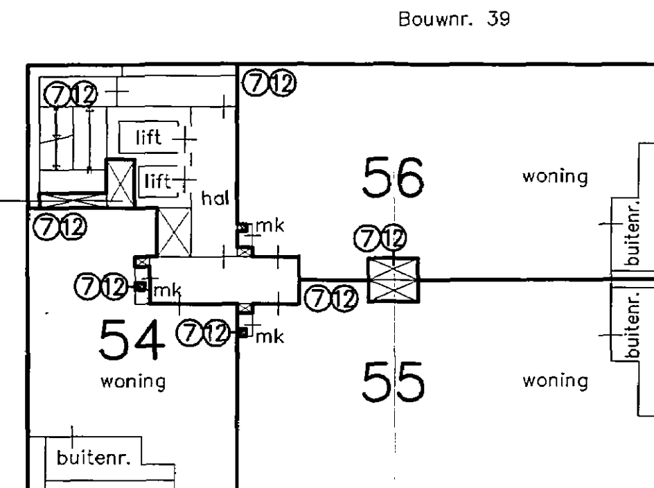
schachten voor algemeen gebruik woningen + comm.ruimten
