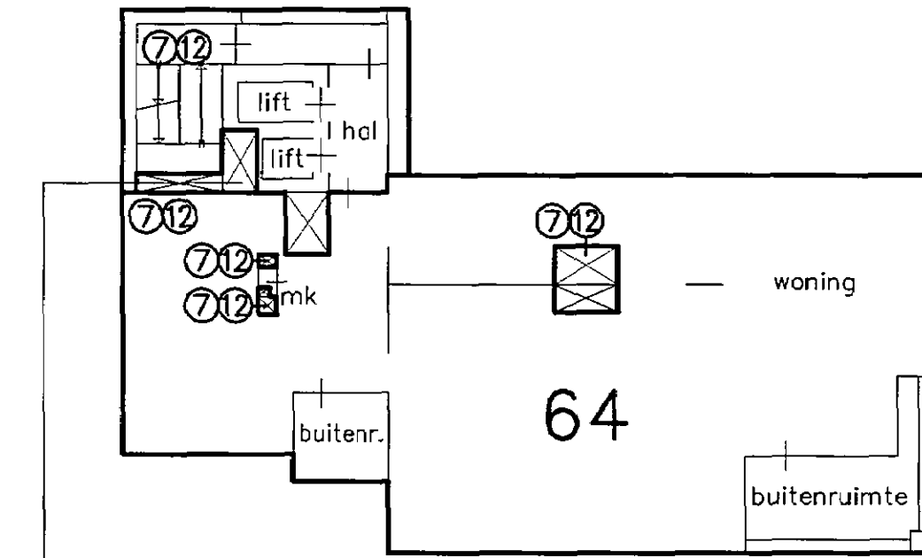
schachten voor algemeen gebruik woningen + comm.ruimten
