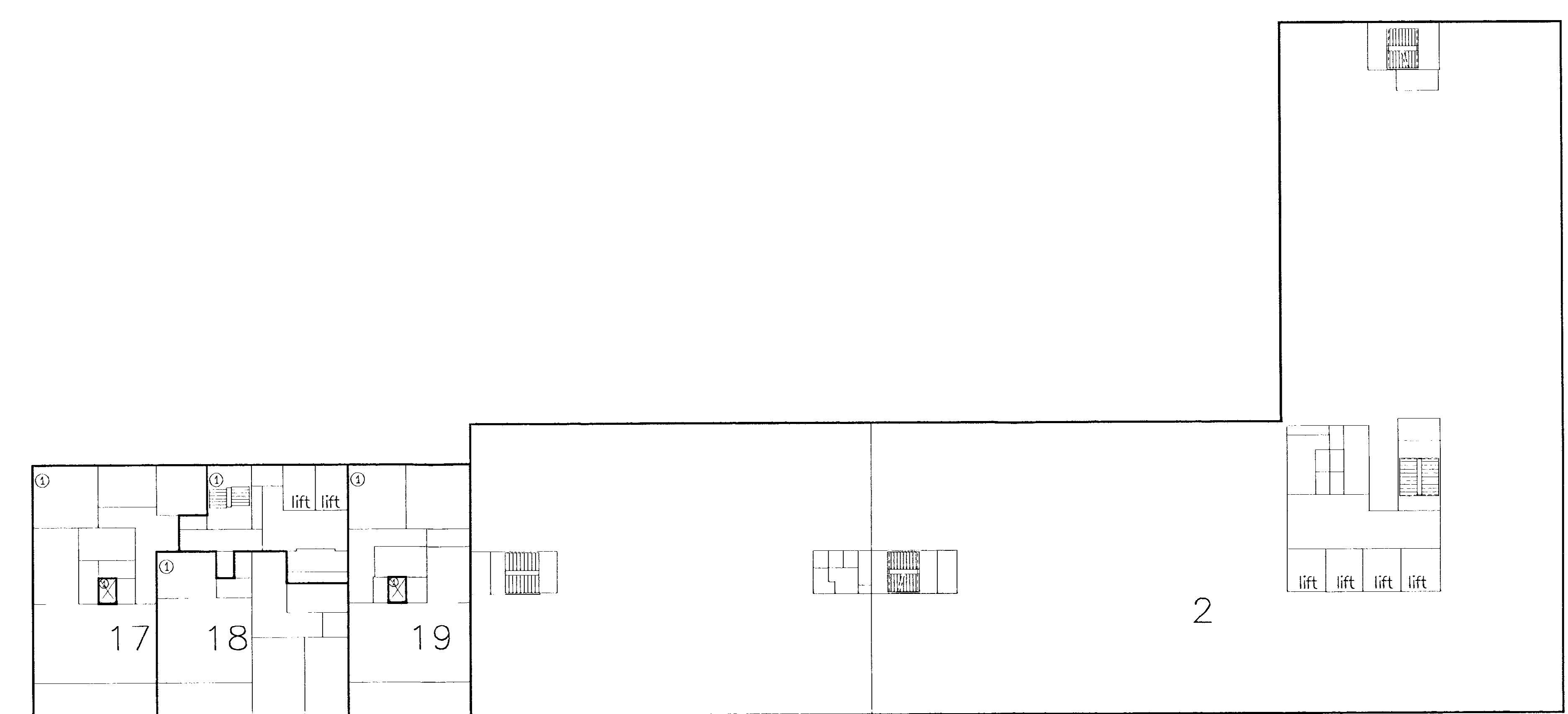
NIVEAU 8 Schaal 1:200
