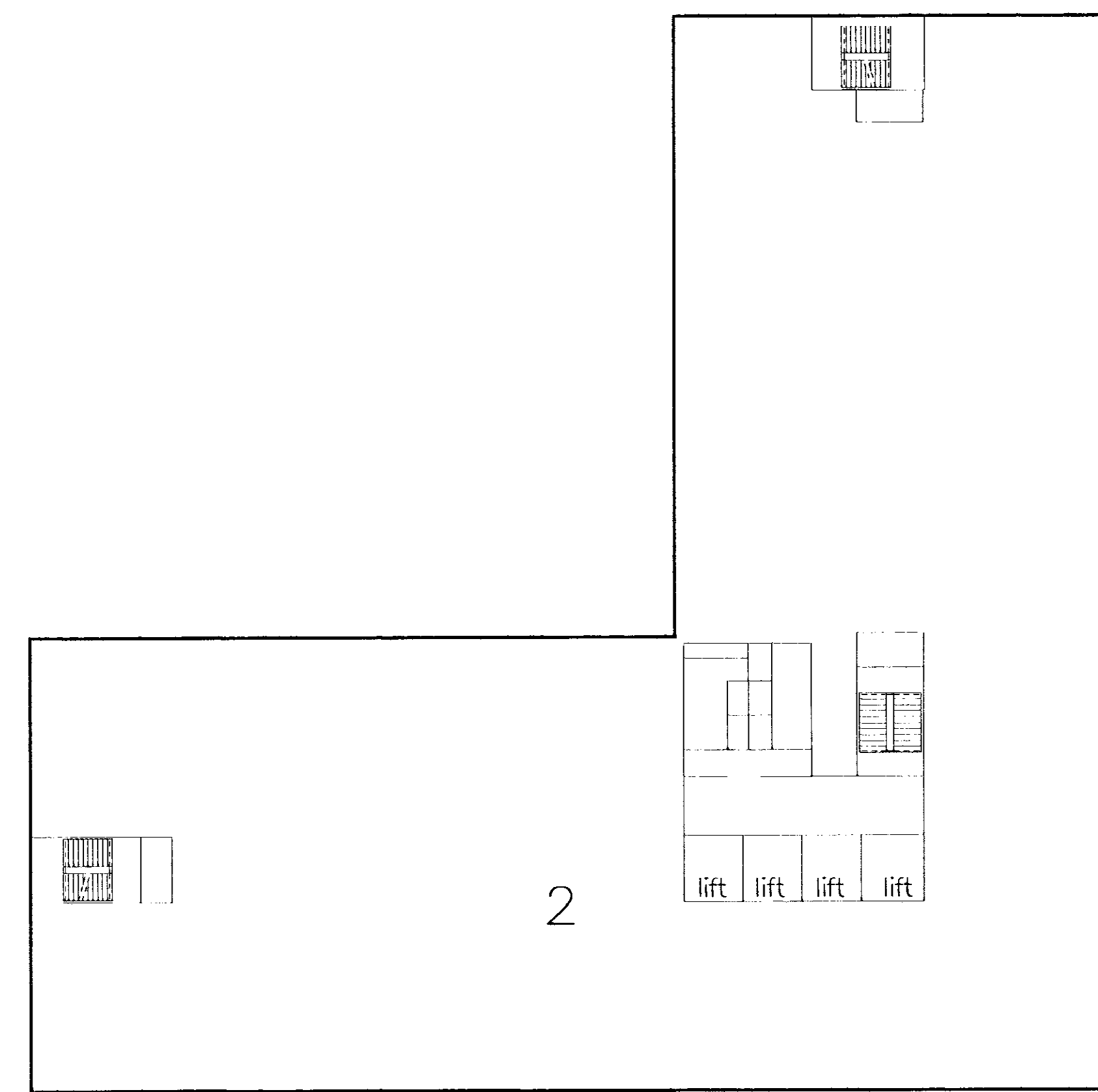
NIVEAU 14 Schaal 1:200
