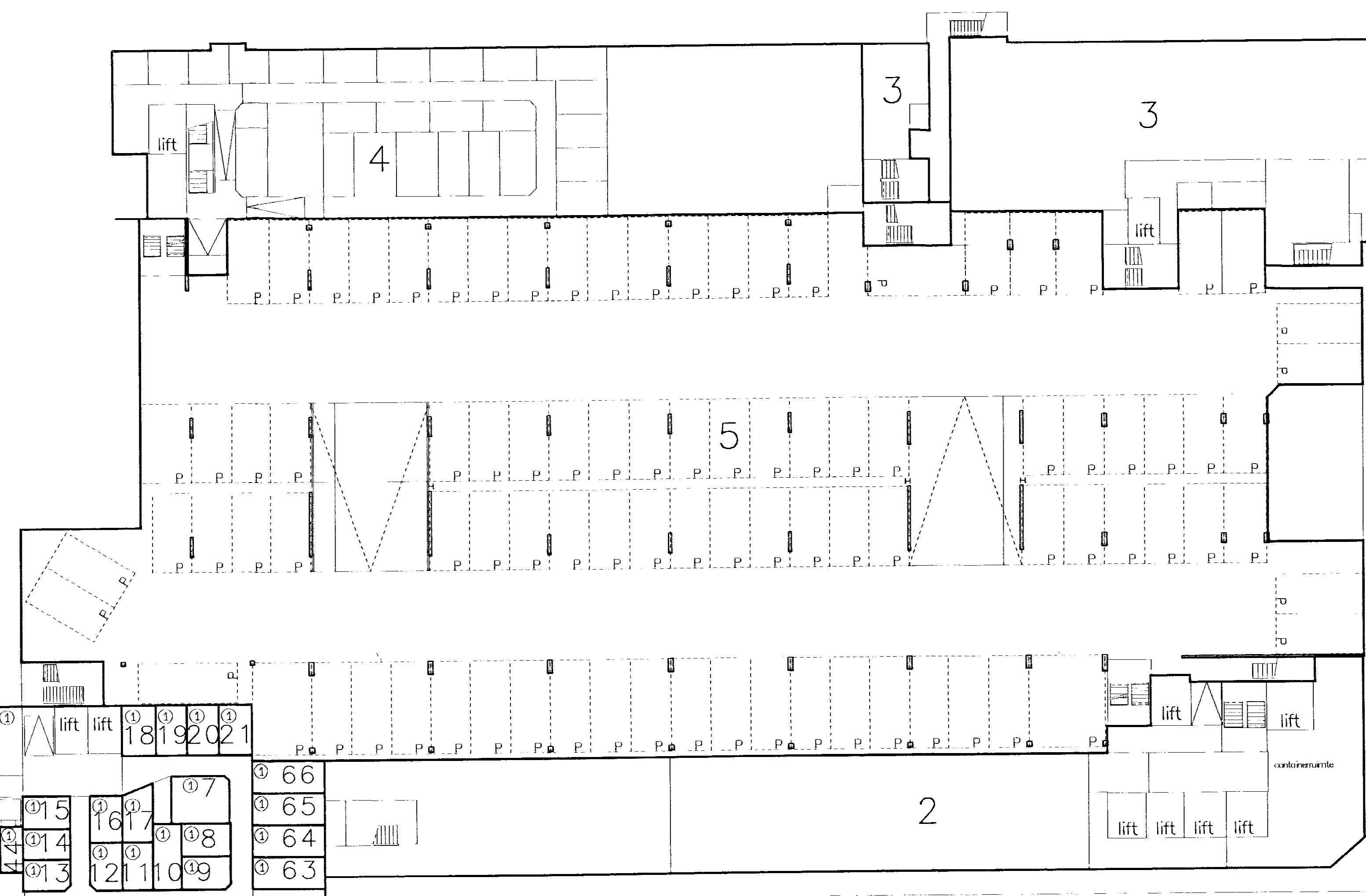
NIVEAU -1 Schaal 1:200
