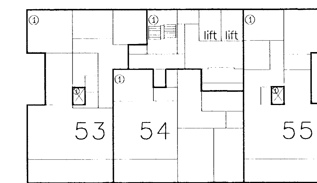
NIVEAU 20 Schaal 1:200
