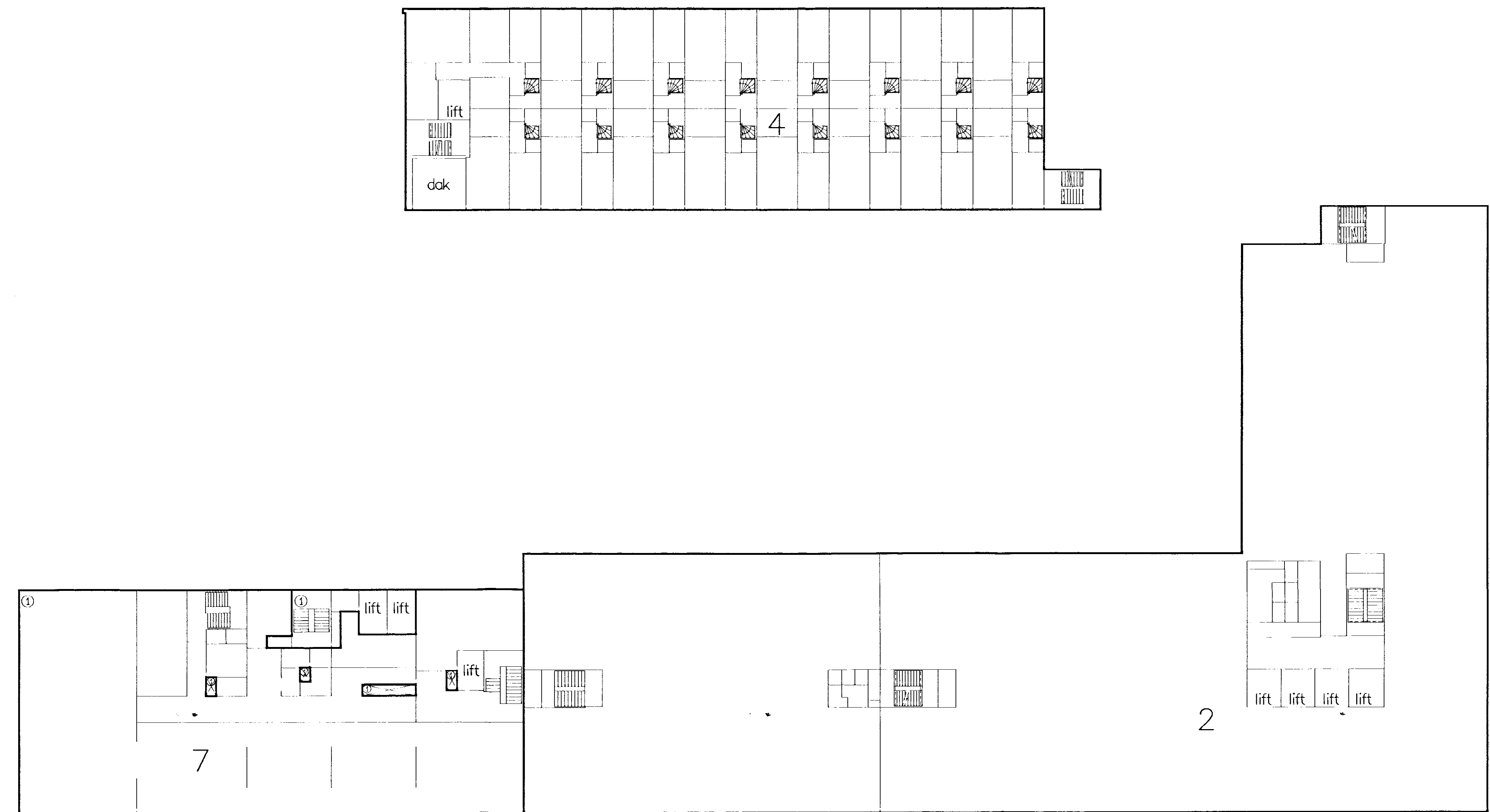
NIVEAU 4 Schaal 1:200
