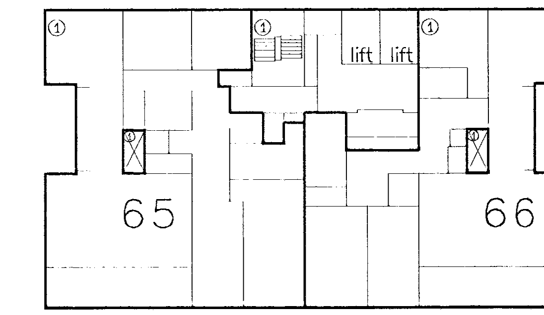
NIVEAU 25 Schaal 1:200
