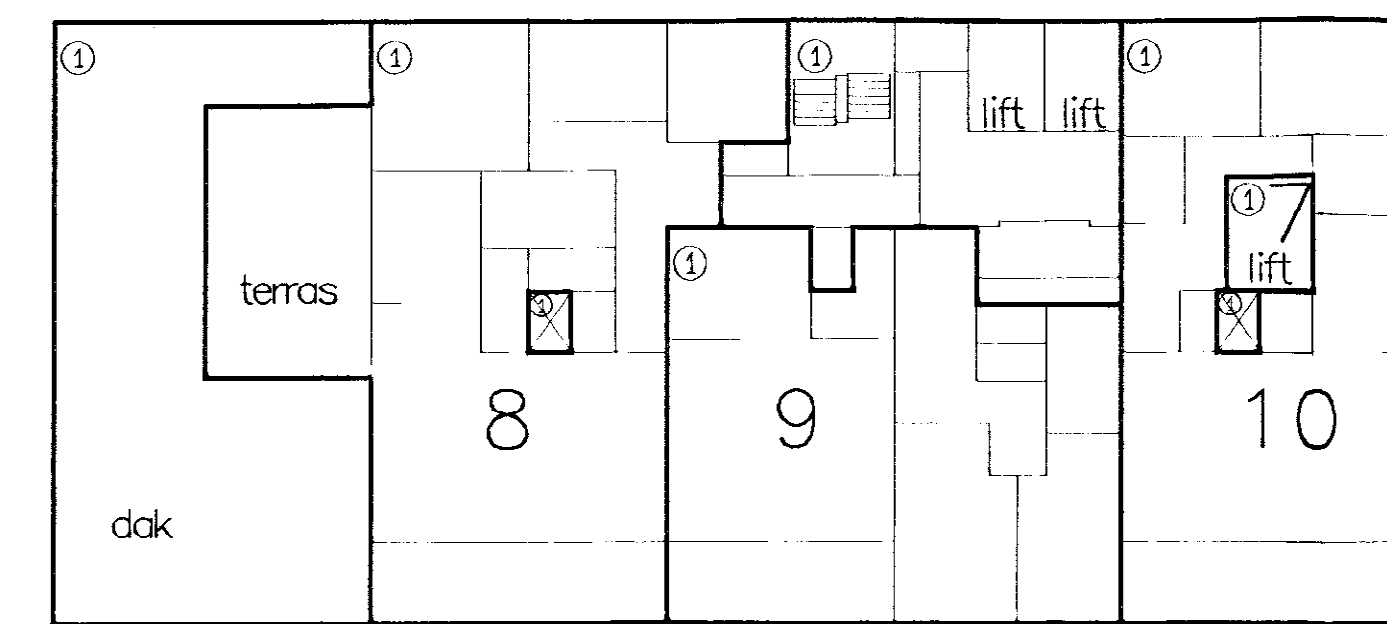
NIVEAU 5 Schaal 1:200
