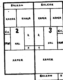
2e verdieping 1 : 200
